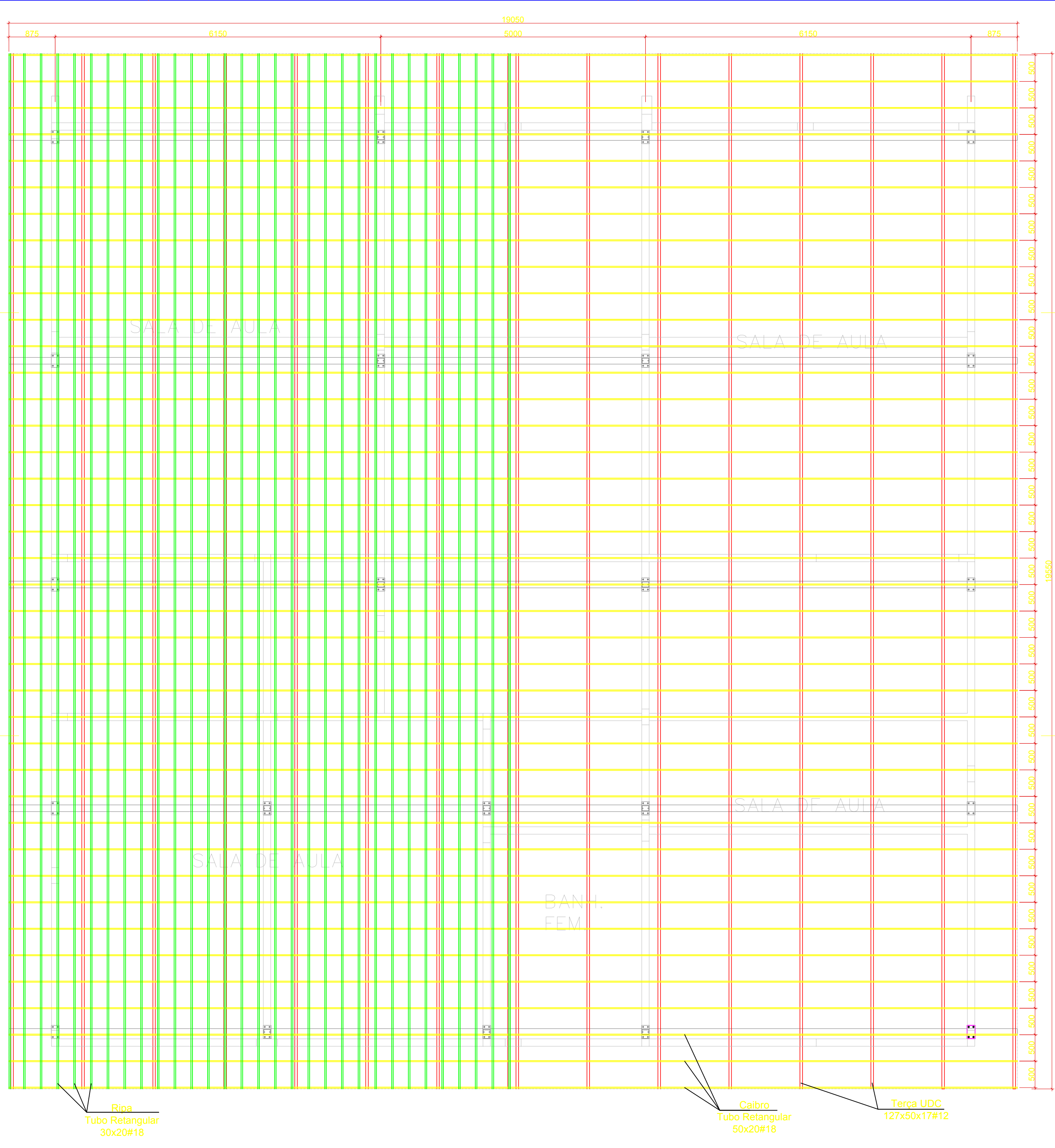
PLANTA DE MONTAGEM - LOCAÇÃO DOS CAIBROS E RIPAS
