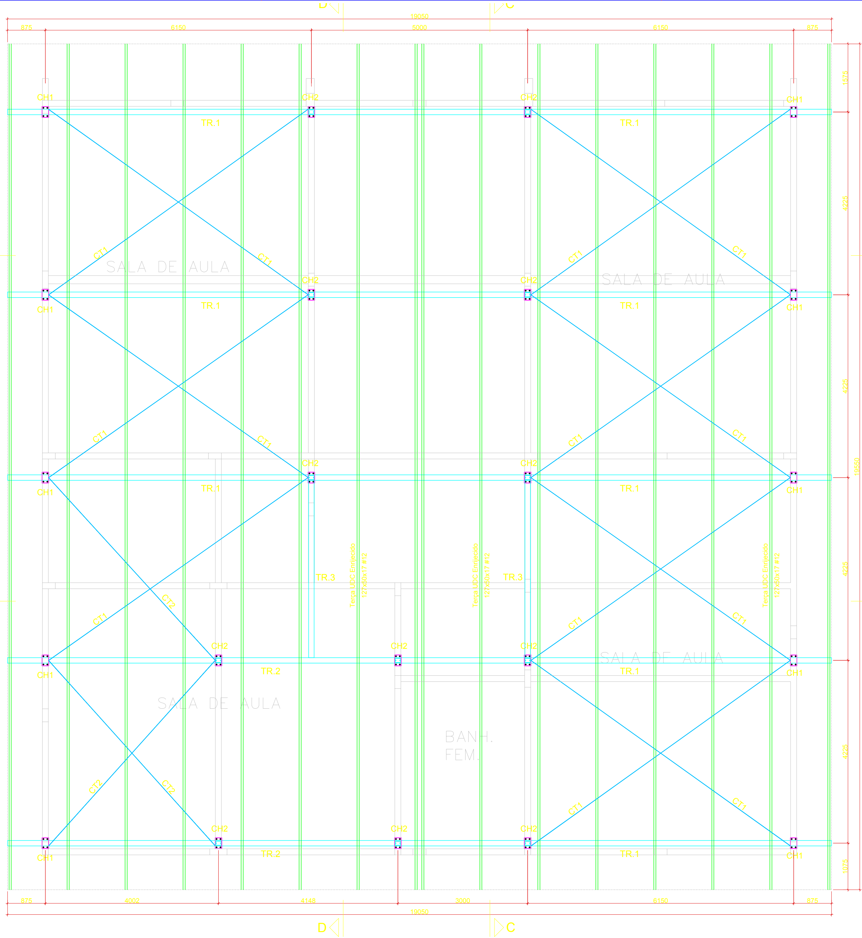
PLANTA DE MONTAGEM - LOCAÇÃO DAS TRELIÇAS, TERÇAS, CONTRAVENTAMENTOS E CHUMBADORES
