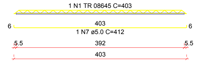
VT5a (10 unidades) (L5) ESC 1:50
