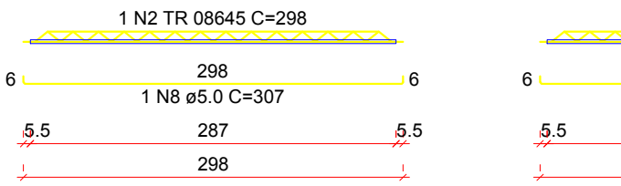
VT9a (9 unidades) (L9) ESC 1:50
