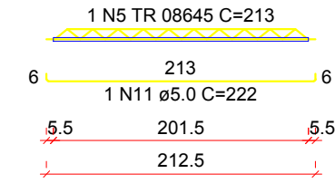
VT14a (13 unidades) (L14) ESC 1:50
