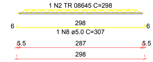
VT15a (7 unidades) (L15) ESC 1:50
