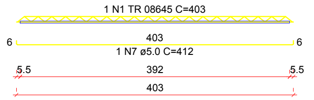
VT6a (12 unidades) (L6) ESC 1:50
