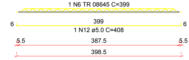
VT16a (12 unidades) (L16) ESC 1:50
