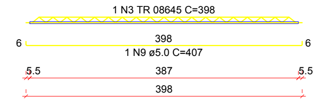
VT11a (12 unidades) (L11) ESC 1:50
