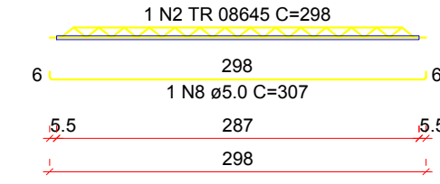
VT8a (3 unidades) (L8) ESC 1:50
