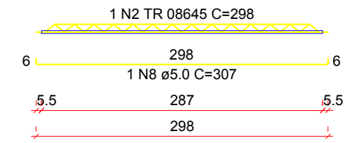
VT10a (13 unidades) (L10) ESC 1:50
