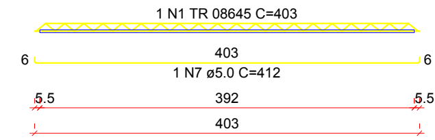
VT3a (12 unidades) (L3) ESC 1:50
