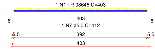
VT4a (12 unidades) (L4) ESC 1:50
