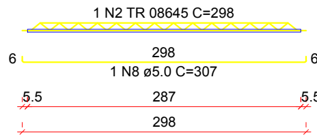
VT7a (7 unidades) (L7) ESC 1:50
