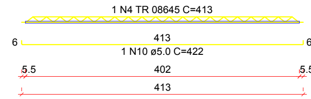
VT12a (12 unidades) (L12) ESC 1:50
