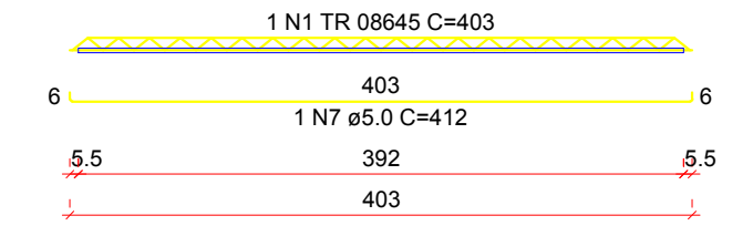
VT1a (12 unidades) (L1) ESC 1:50
