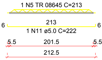
VT13a (5 unidades) (L13) ESC 1:50
