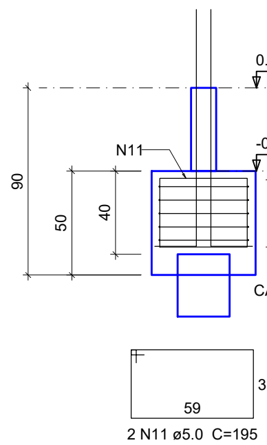
CORTE ESC 1:25
