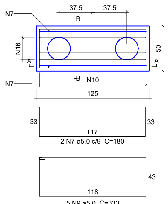
B207 2xD25 C=5M PLANTA ESC 1:25
