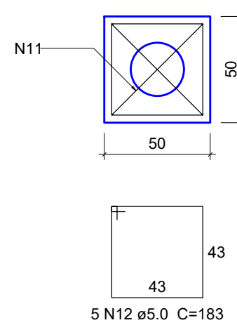
B210 1xD25 C=5M PLANTA ESC 1:25
