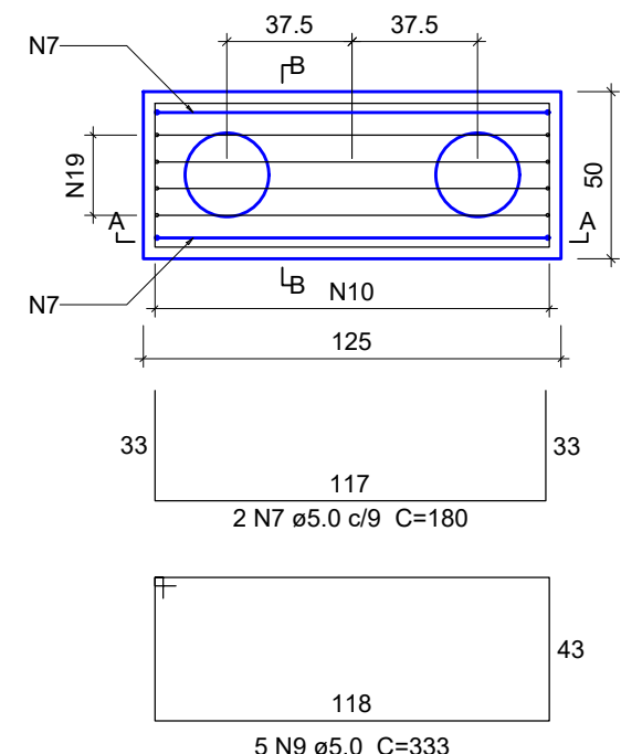
B206 2xD25 C=5M PLANTA ESC 1:25
