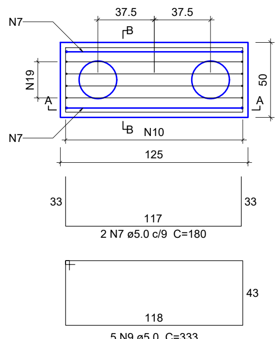
B214 2xD25 C=5M PLANTA ESC 1:25
