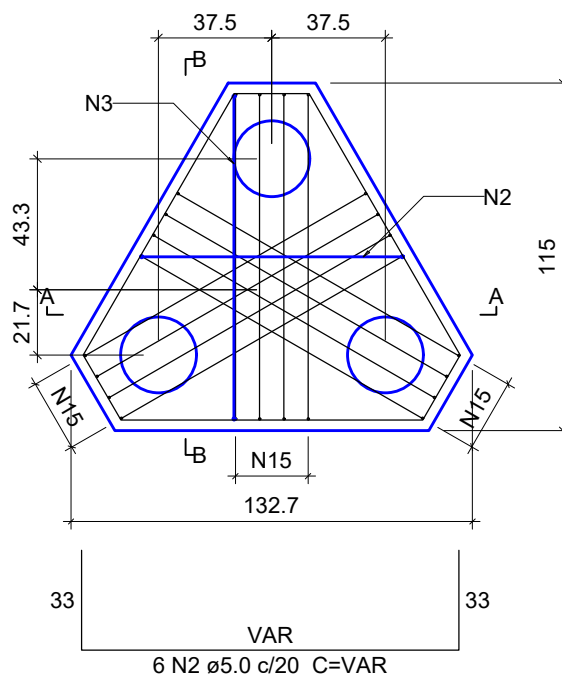
B185 3xD25 C=2M PLANTA ESC 1:25
