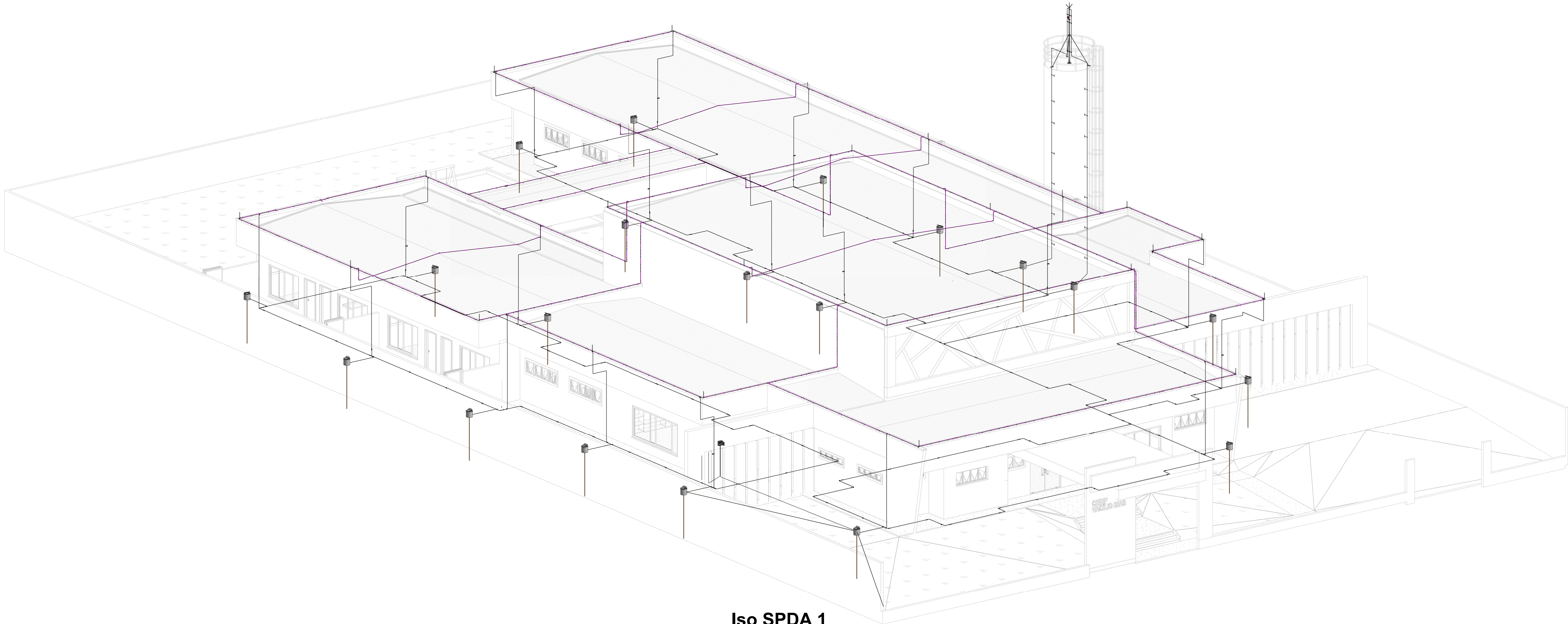
Iso SPDA 1
