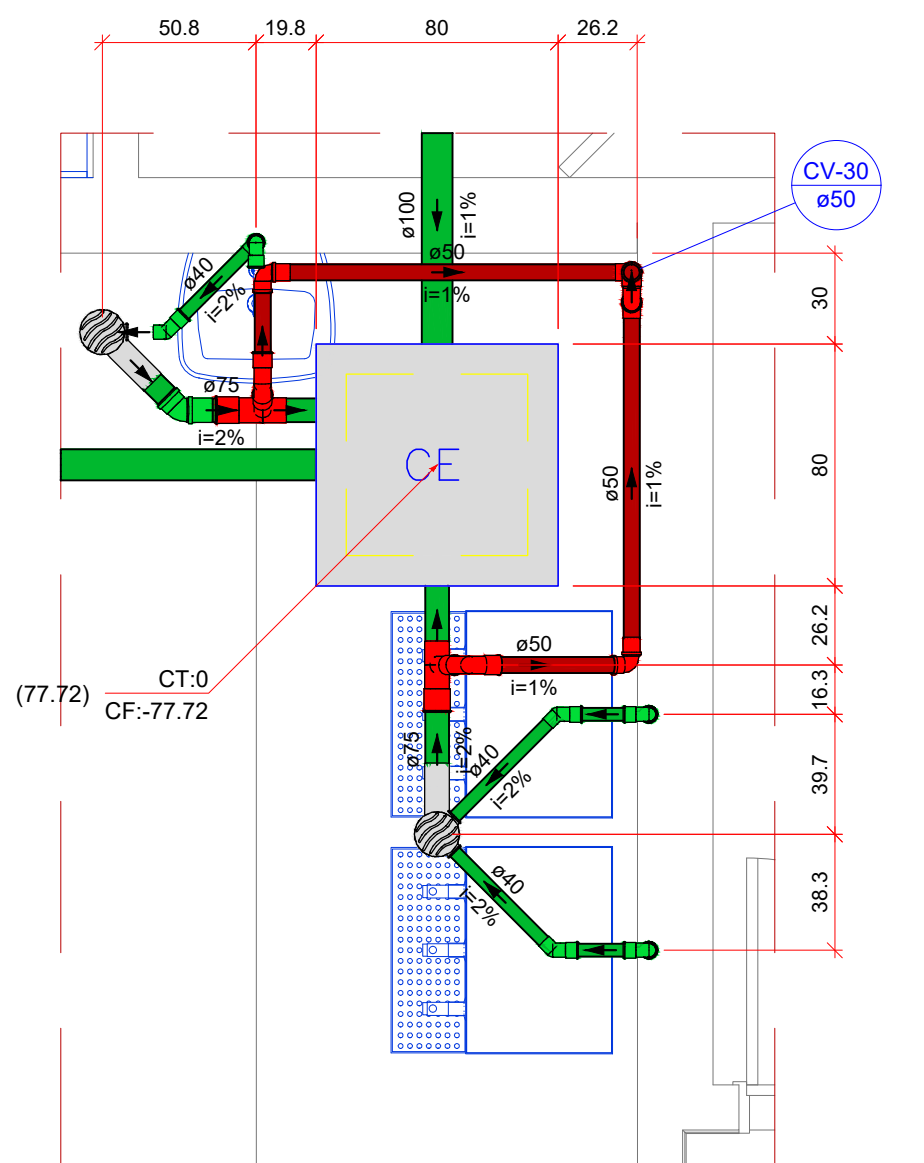
Detalhe S9 Escala 1:25
