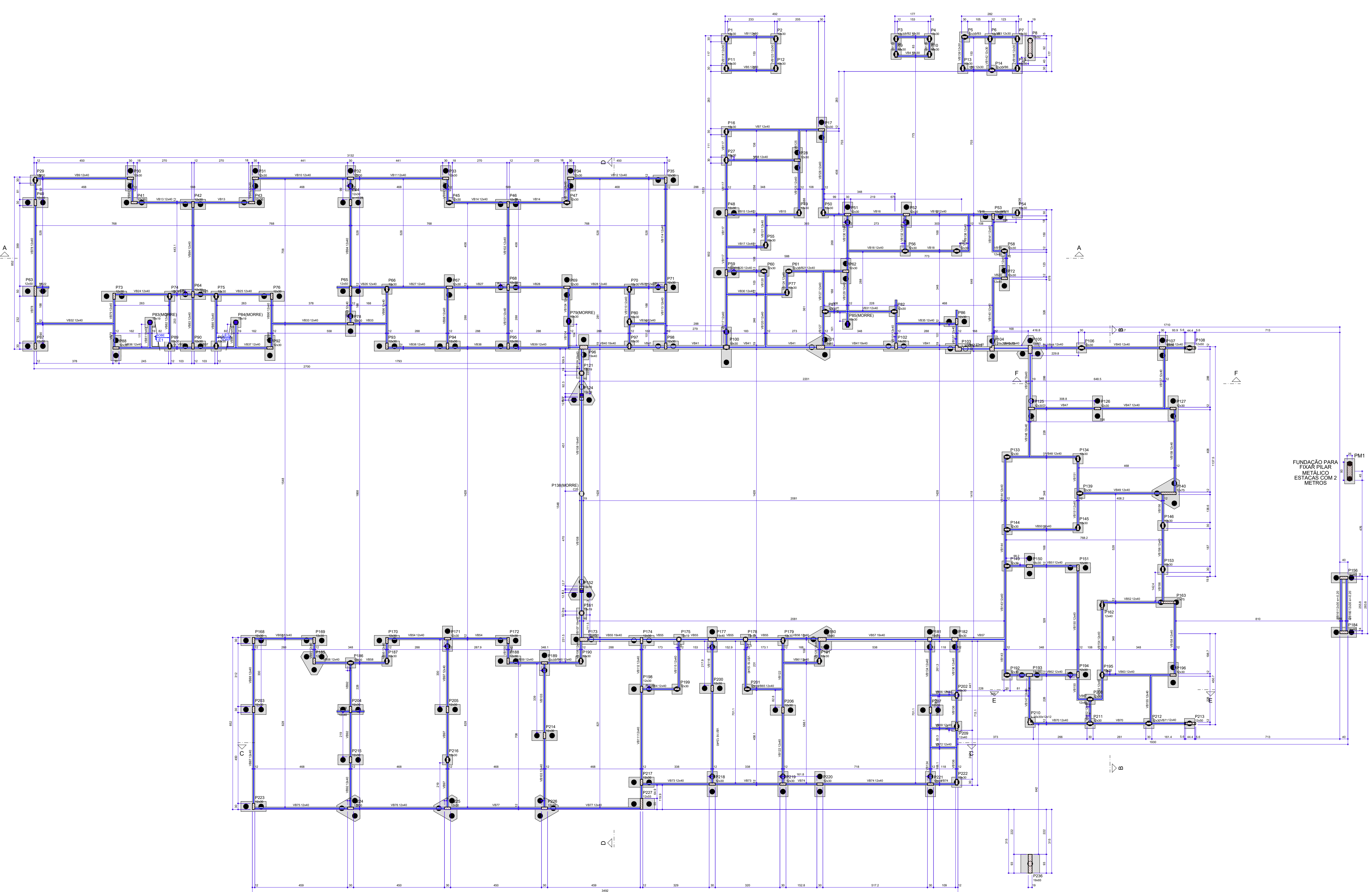
Forma do pavimento TÉRREO (Nível 0.15) escala 1:75
